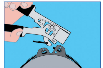
4. Überschüssiges Band abschneiden
