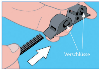
1. Band in den Verschluss einführen
